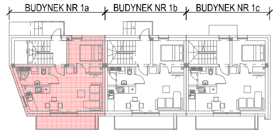
RZUT PARTERU
