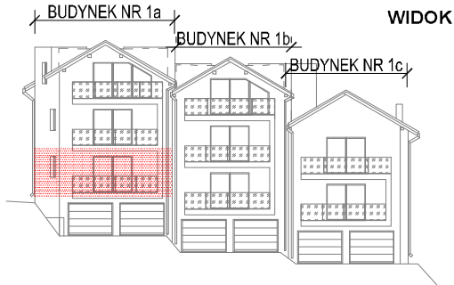
ELEWACJA POŁUDNIOWA
