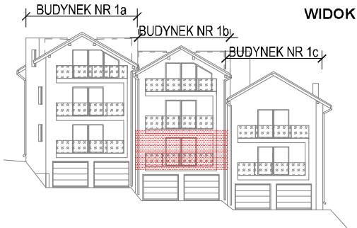
ELEWACJA POŁUDNIOWA
