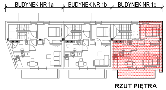
RZUT PIĘTRA
